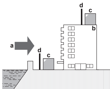
a Seewind b Gebäude c Außeneinheit d Windschutz
