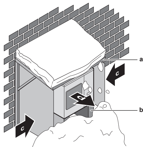
a Schneeabdeckung oder Unterstand b Unterstell (Mindesthöhe = 150 mm) c Vorherrschende Windrichtung d Luftauslass
