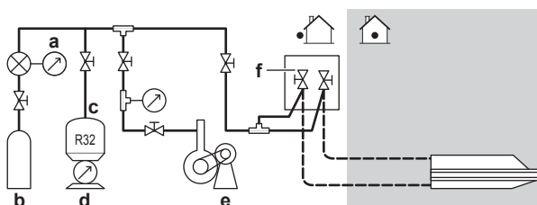
a Druckmesser b Stickstoff c Kältemittel d Wiegevorrichtung e Vakuumpumpe f Absperrventil
