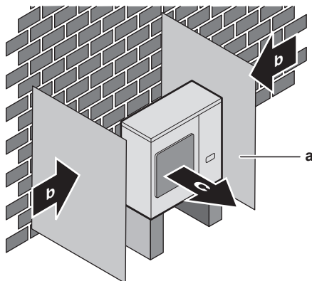
a Ablenkplatte b Vorherrschende Windrichtung c Luftauslass
