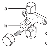
a Apertura di servizio e coperchio dell'apertura di servizio b Stelo della valvola c Collegamento delle tubazioni esistenti
