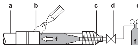
a Tubazione del refrigerante b Parte da brasare c Nastratura d Valvola manuale e Valvola per la riduzione della pressione f Azoto
