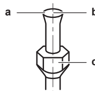
a La superficie interna della svasatura DEVE essere priva di difetti. b L'estremità del tubo DEVE essere svasata in modo uniforme in un cerchio perfetto. c Assicurarsi che il dado svasato sia installato.
