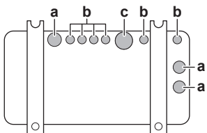
a Foro di scolo. Installare un tappo di scarico (2). b Foro di scolo. Installare un tappo di scarico (1). c Foro di scolo per presa di drenaggio
