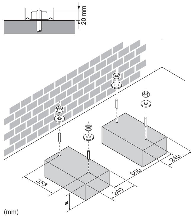
a 100 mm über erwartbarer Schneehöhe
