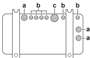
a Orifice de drainage. Installez le bouchon de drainage (2). b Orifice de drainage. Installez le bouchon de drainage (1). c Orifice de drainage pour raccord de drainage
