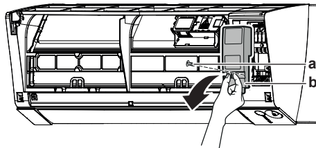
a Vite del coperchio di servizio
