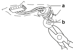
a Schutzhülse b Clip
