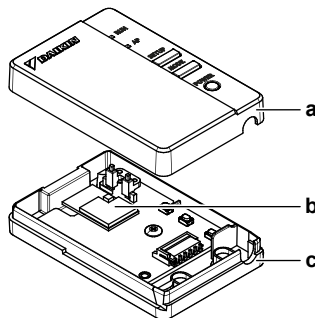
a Oberes Gehäuseteil b Platine des WLAN-Adapters c Unteres Gehäuseteil
