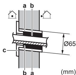
a In die Wand einzubettendes Rohr
