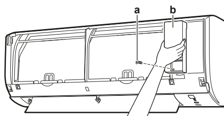
a Schraube von Wartungsblende b Wartungsblende
