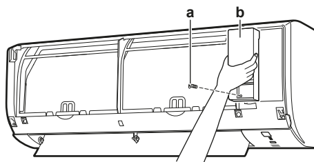
a Vite del coperchio di servizio
