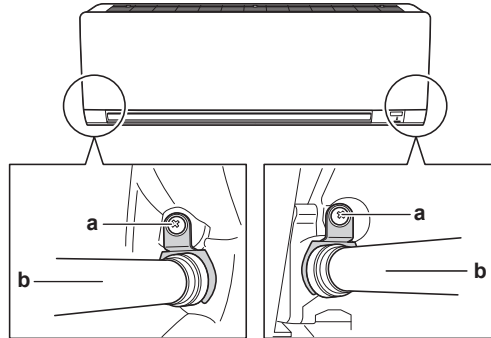
a Befestigungsschraube der Isolation b Abflussschlauch
