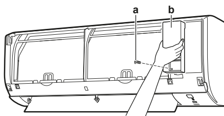
a Vite del coperchio di servizio
