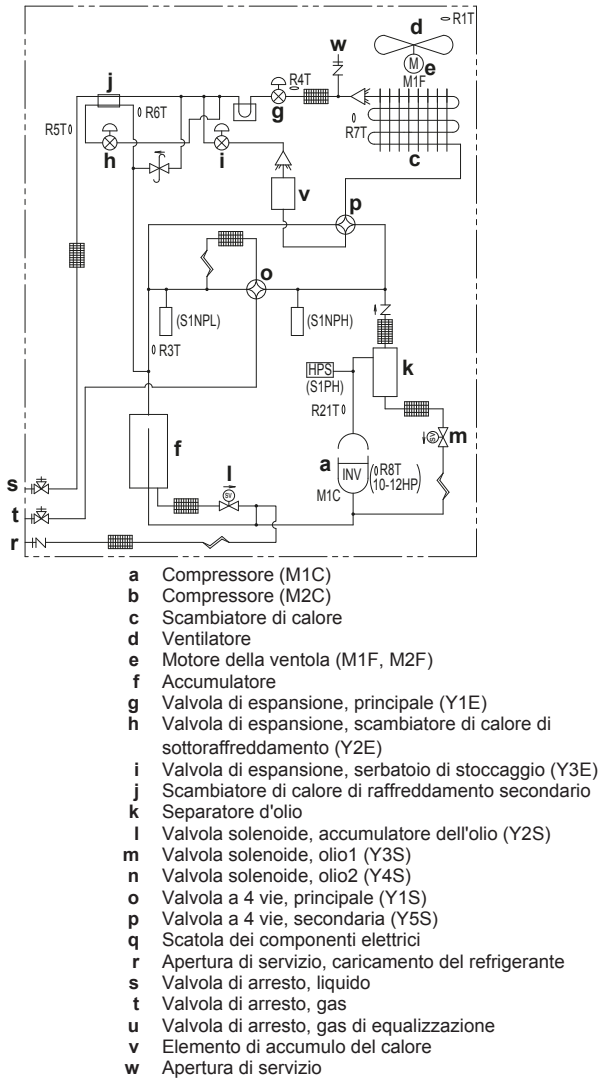
Schema delle tubazioni: RYYQ8~12
