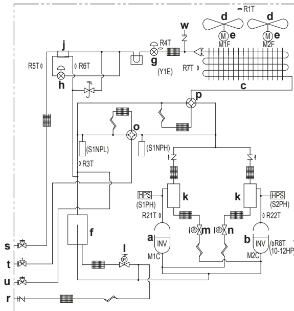
Schema delle tubazioni: RYMQ14~20
