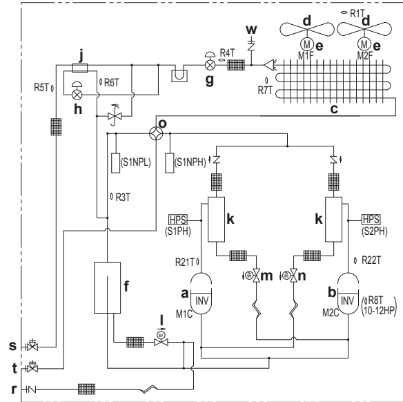
Schema delle tubazioni: RXYQ14~20
