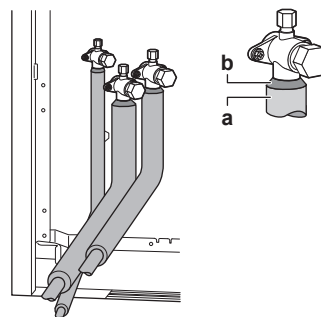
a Materiale di isolamento b Calafataggio, ecc.
