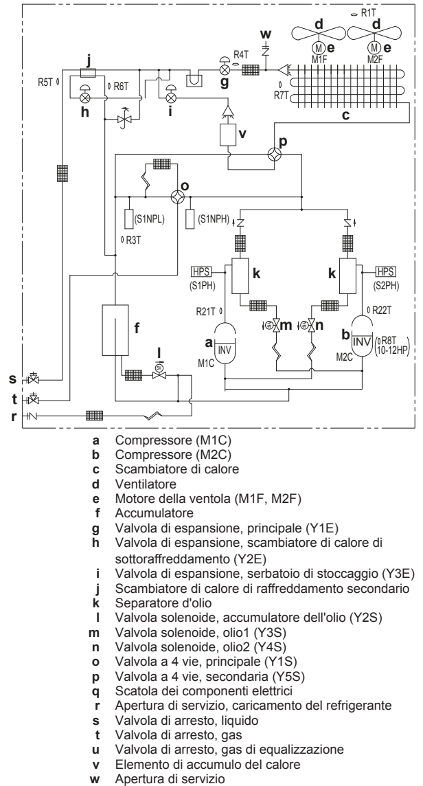
Schema delle tubazioni: RYYQ14~20
