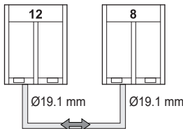
Seul le tuyau de compensation est illustré
