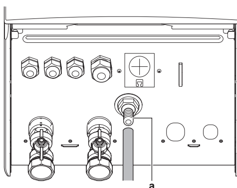
a Connettore della bacinella di drenaggio
