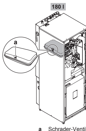
a Schrader-Ventil
