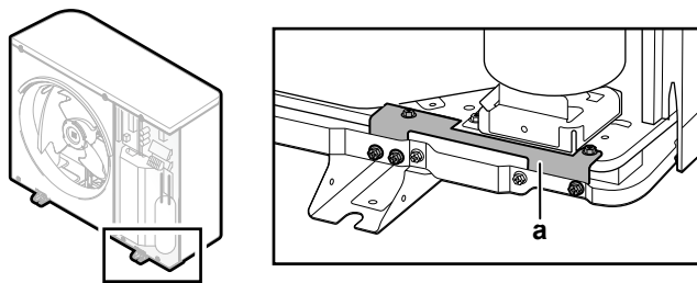
a Supporto per il trasporto
