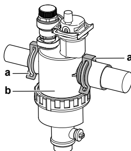
a Fermaglio b Filtro magnetico/separatore di sporizia
