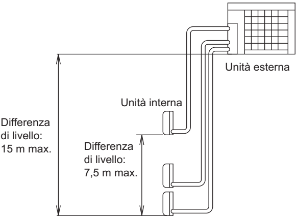
Unità esterna posta più in alto delle unita interne.
