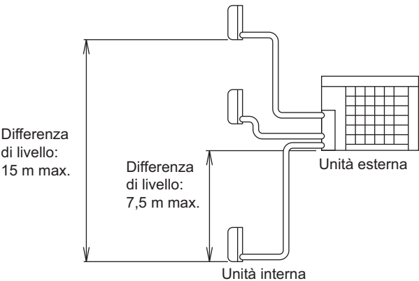
Unità esterna posta diversamente. (Più bassa di una o più unità interne).
