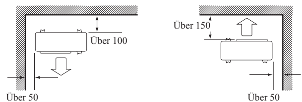
Draufsicht
