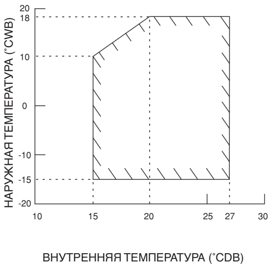
ОБОГРЕВ
