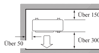
Draufsicht
