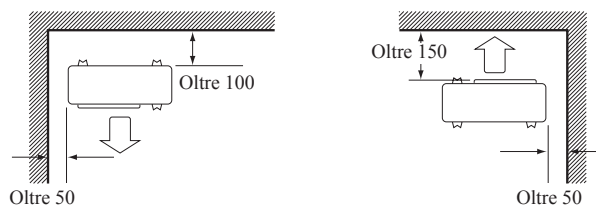
Vista superiore
