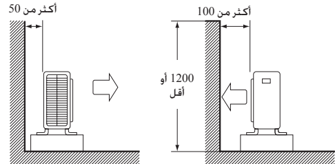
منظر جانبي
