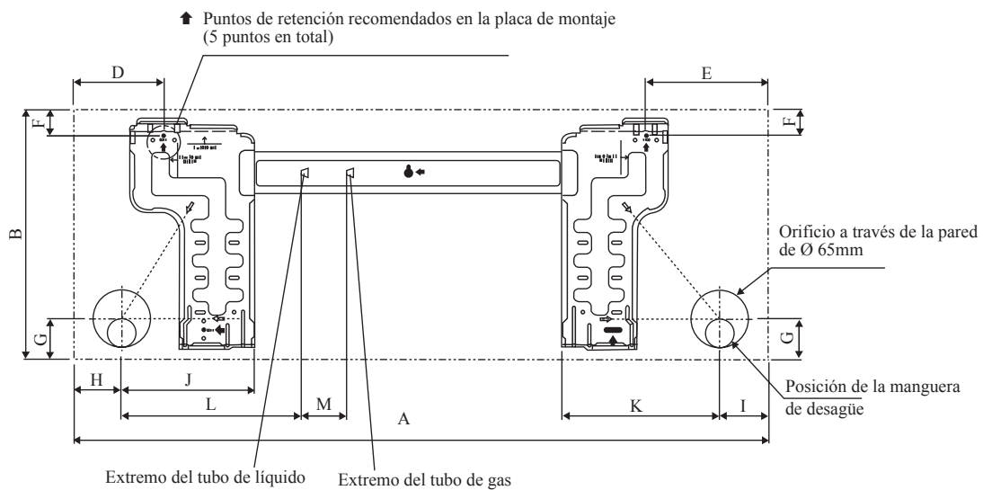
ALTERNATIVA DE LA PLACA BASE 25/35
