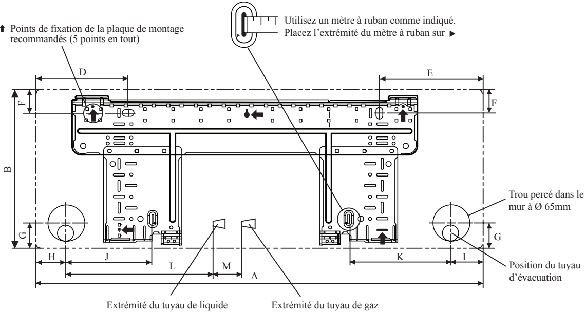
PLAQUE D'INSTALLATION 25/35
