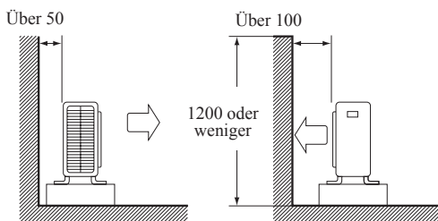
Seitenansicht
