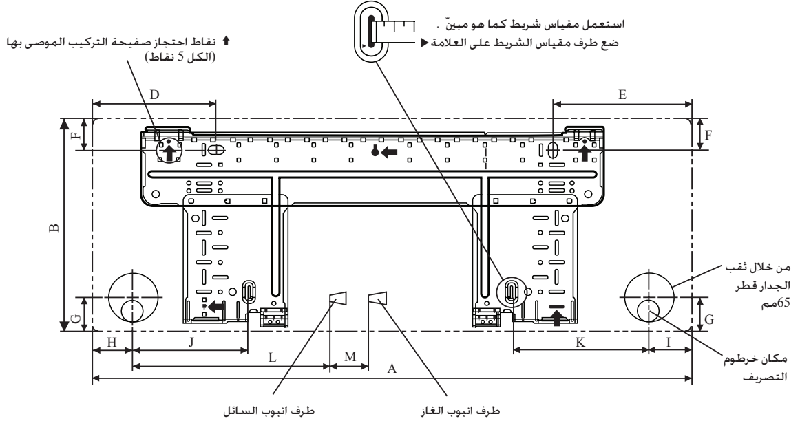
لوحة التركيب 25/35
