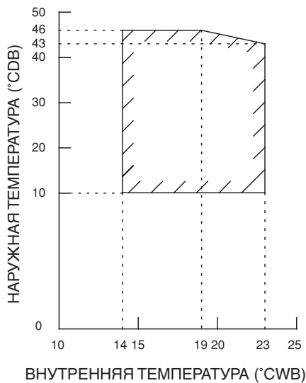
ОХЛАЖДЕНИЕ
