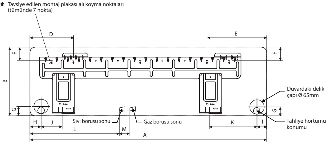
KURULUM LEVHASI 50/60
