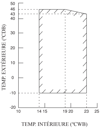
REFROIDISSEMENT
