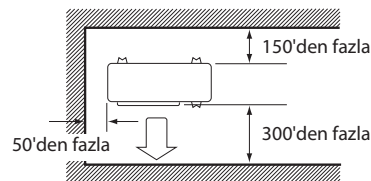
Yukarıdan Görünüm
