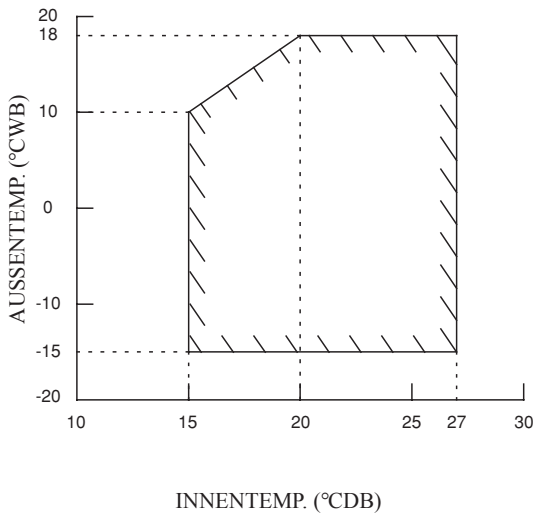
HEIZEN
