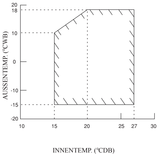
HEIZEN
