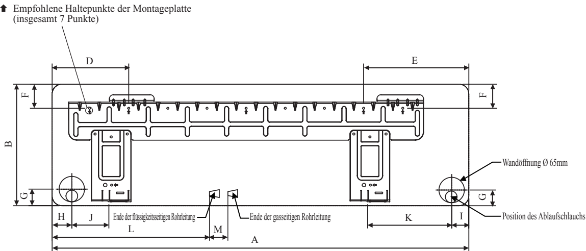
MONTAGEPLATTE 50/60
