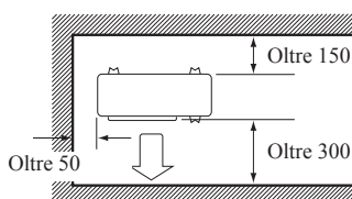
Vista superiore
