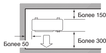
Вид сверху
