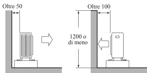
Vista laterale
