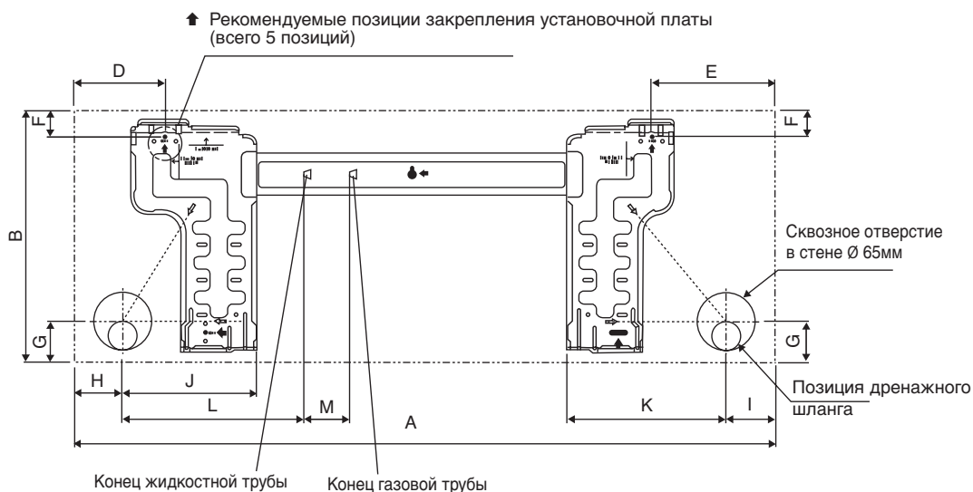
АЛЬТЕРНАТИВНЫЙ ВАРИАНТ УСТАНОВКИ ПЛАСТИНА 25/35
