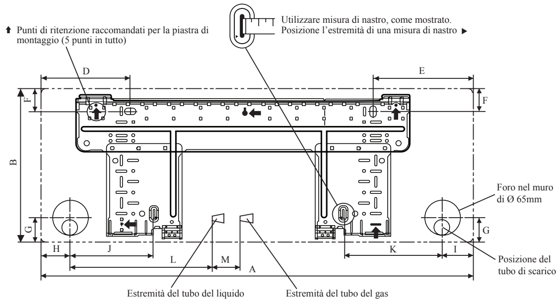
LASTRA DI INSTALLAZIONE 25/35
