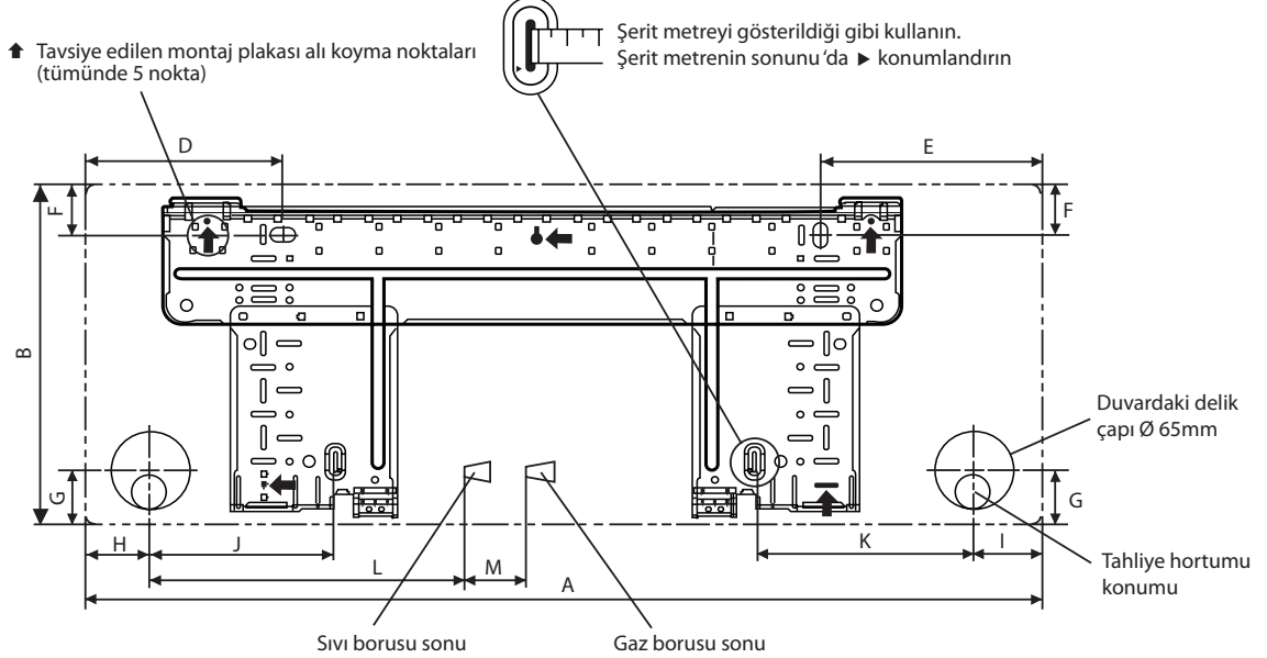
KURULUM LEVHASI 25/35
