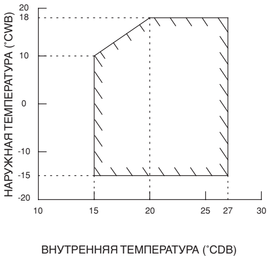
ОБОГРЕВ
