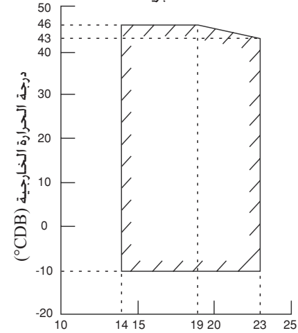
التبريد
