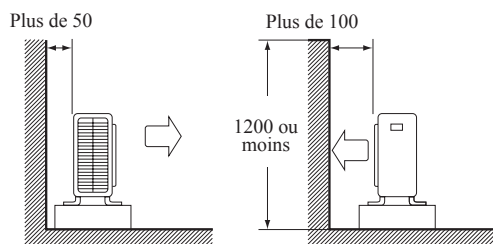
Vue latérale
