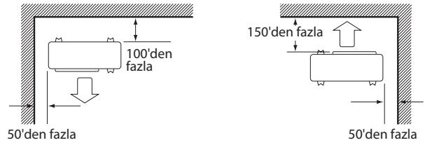
Yukarıdan Görünüm
