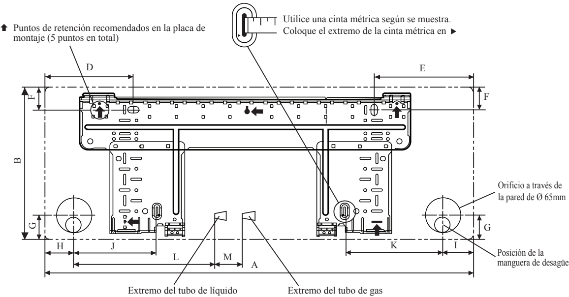
PLACA DE INSTALACIÓN 25/35
