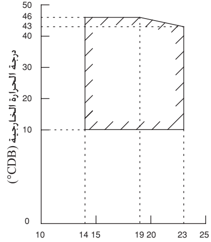
التبريد
