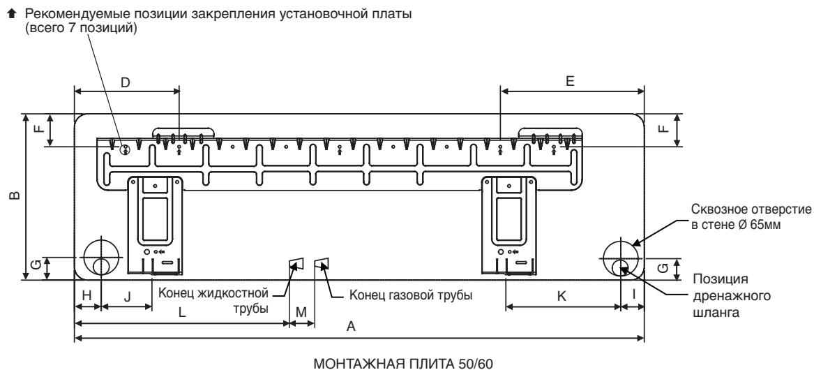
МОНТАЖНАЯ ПЛИТА 50/60
