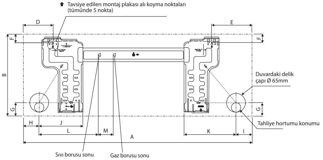
ALTERNATIF YÜKLEME PLAKASI 25/35
