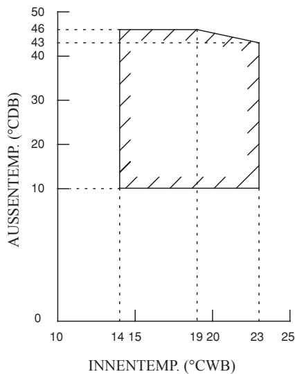
KÜHLUNG
