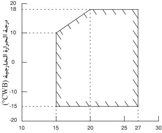
التدفئة
