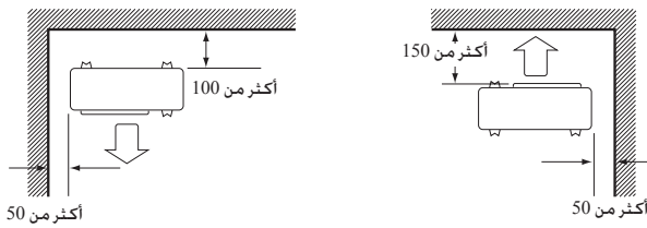
منظر علوي
