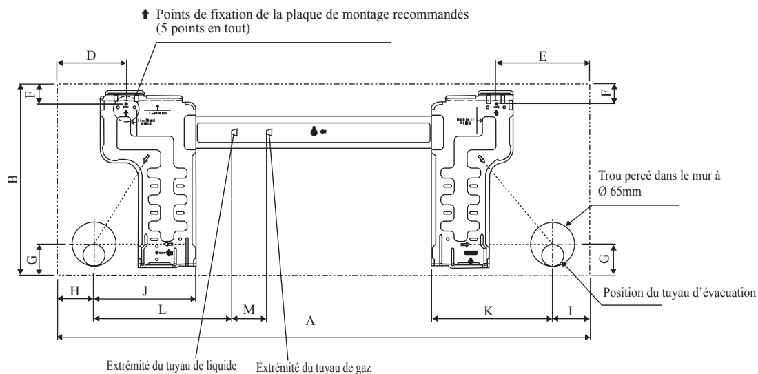
ALTERNATIVE PLAQUE D'INSTALLATION 25/35
