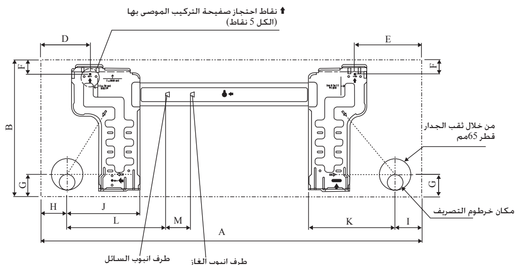
تركيب اللوحة (البديلة) 25/35
