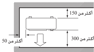
منظر علوي
