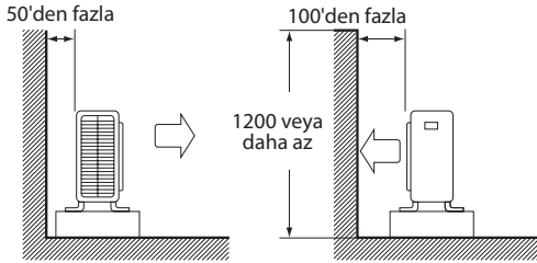
Yandan Görünüm
