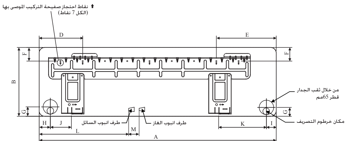
لوحة التركيب 50/60
