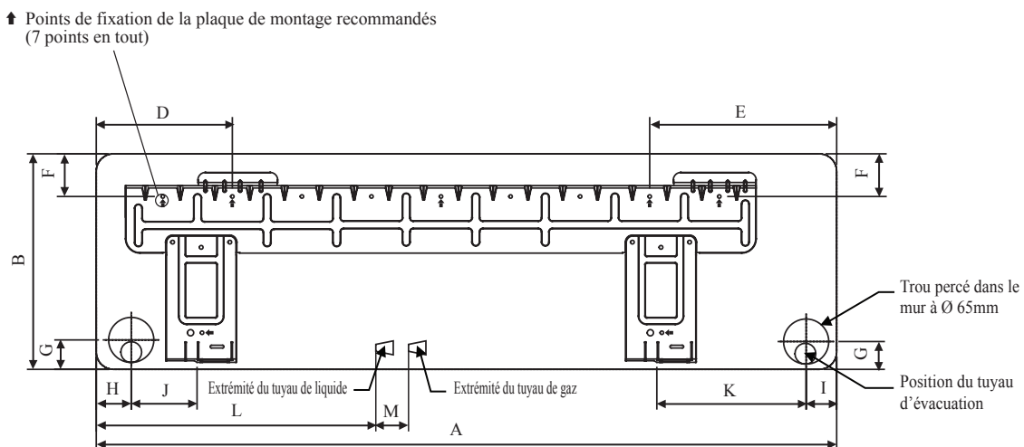
PLAQUE D'INSTALLATION 50/60
