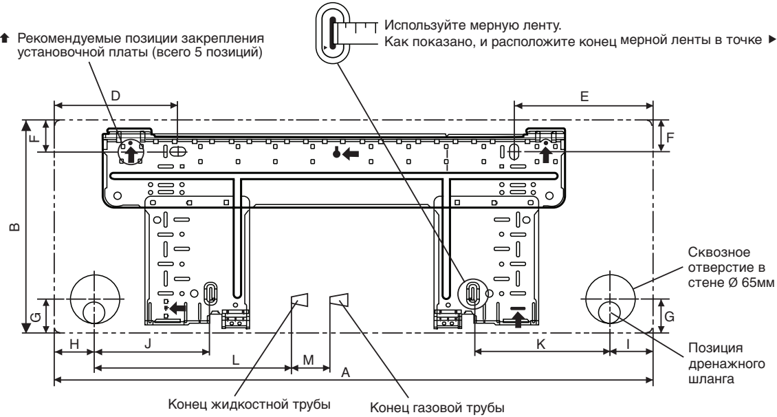
МОНТАЖНАЯ ПЛИТА 25/35
