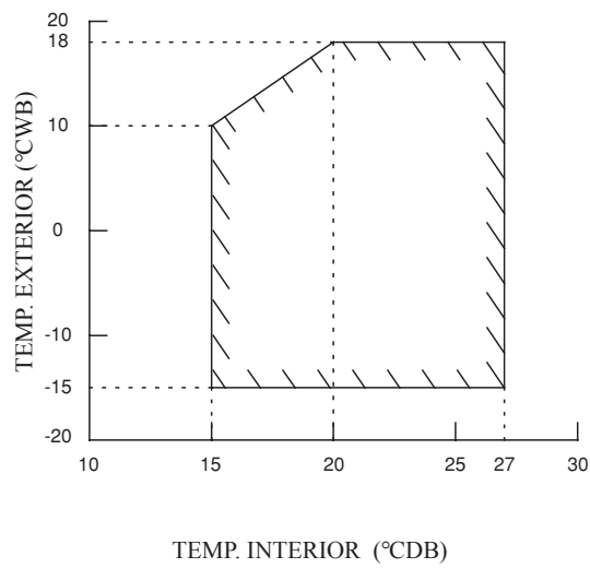
CALEFACCIÓN
