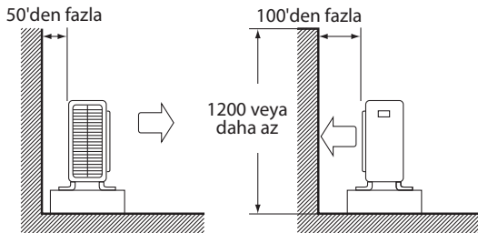
Yandan Görünüm
