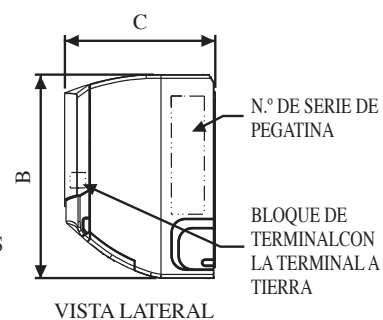
VISTA LATERAL
