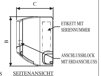
SEITENANSICHT
