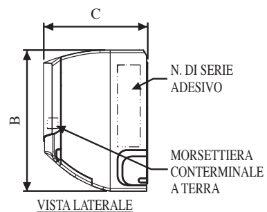
VISTA LATERALE
