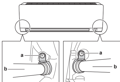
a Vite di fissaggio dell'isolante b Tubo flessibile di drenaggio
