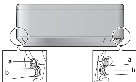
a Vis de fixation d'isolation b Tuyau de vidange
