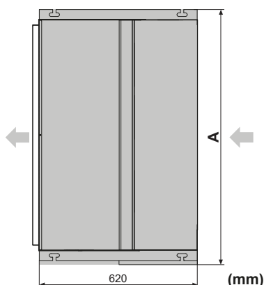
12-1 Dimensioni dell'apertura nel controsoffitto (A)
