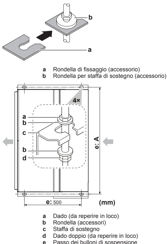
12-2 Interasse dei tiranti di sospensione (A)
