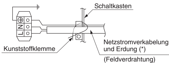
HINWEIS 1: Detail der Klemmleiste für Starkstrom
