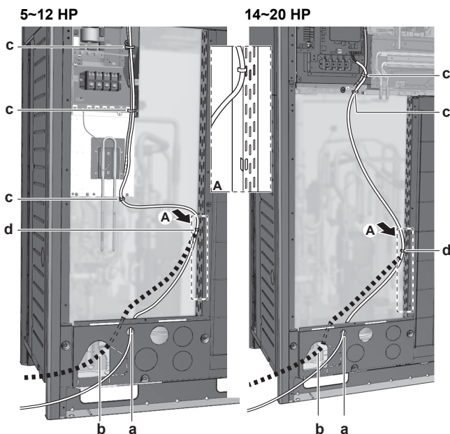
a Verbindungskabel (Möglichkeit 1) (a)
