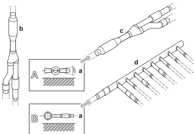
a Superficie orizzontale b Giunti Refnet montati verticalmente c Giunti Refnet montati orizzontalmente d Collettore
