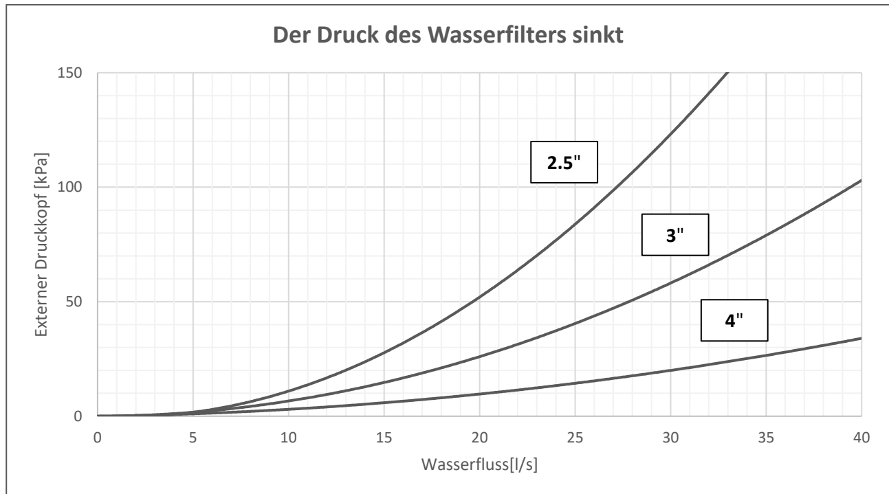
Abb. 13 – Druckabfall des Wasserfilters
