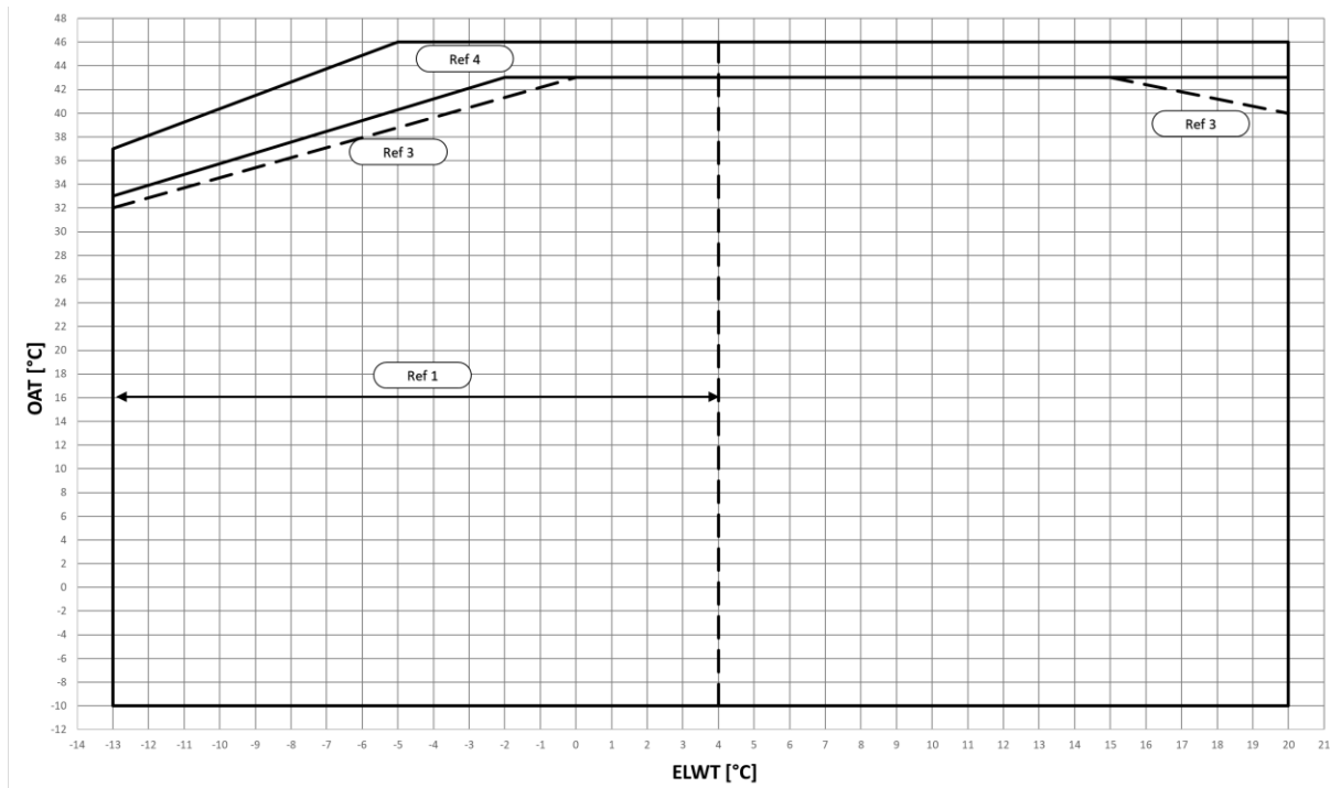
Fig. 11 - EWYTx5B-S Limites opérationnelles du mode refroidissement
