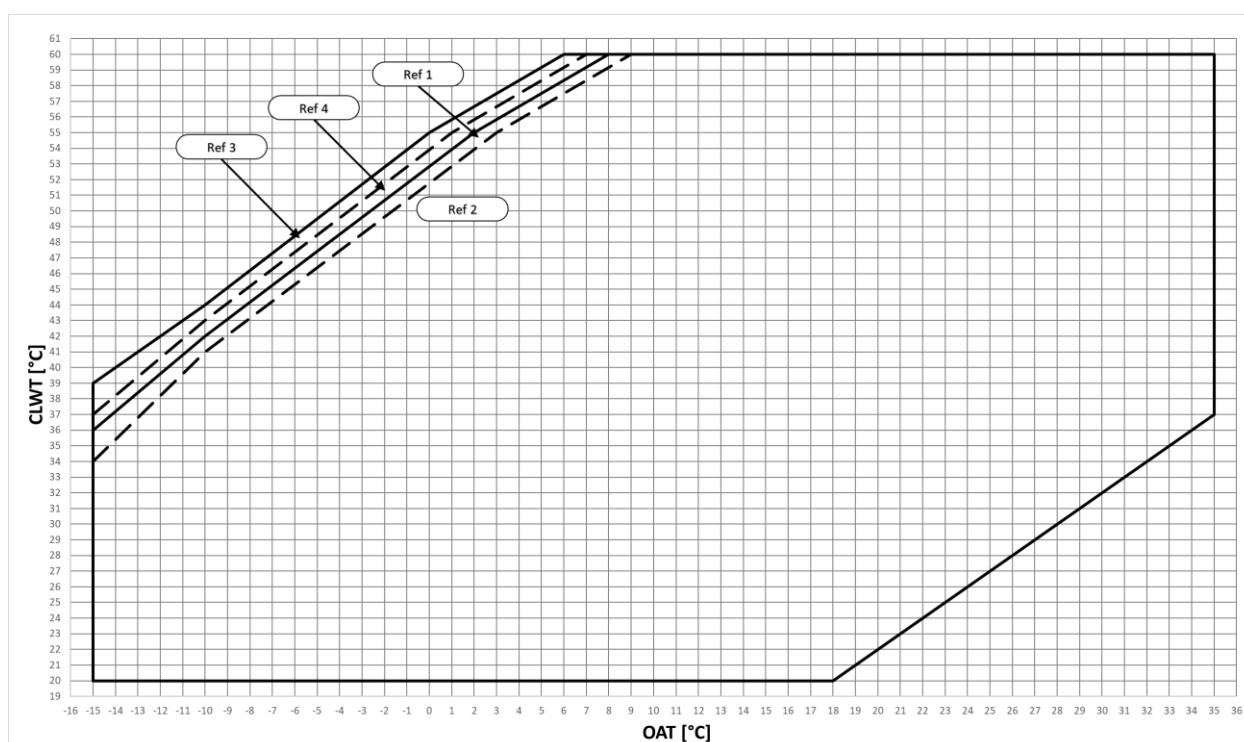
Fig. 16 - EWYT~B-X Limites opérationnelles du mode chauffage
