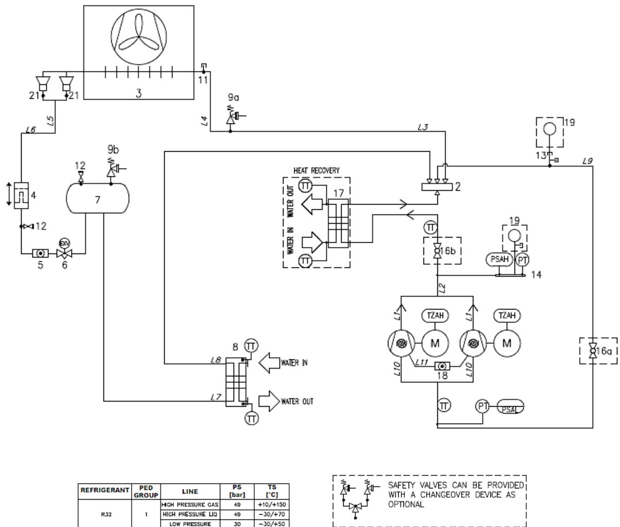
Fig. 17 - Schéma de tuyauterie de réfrigérant EWYTx5B d'une unité à circuit unique (P&ID)
