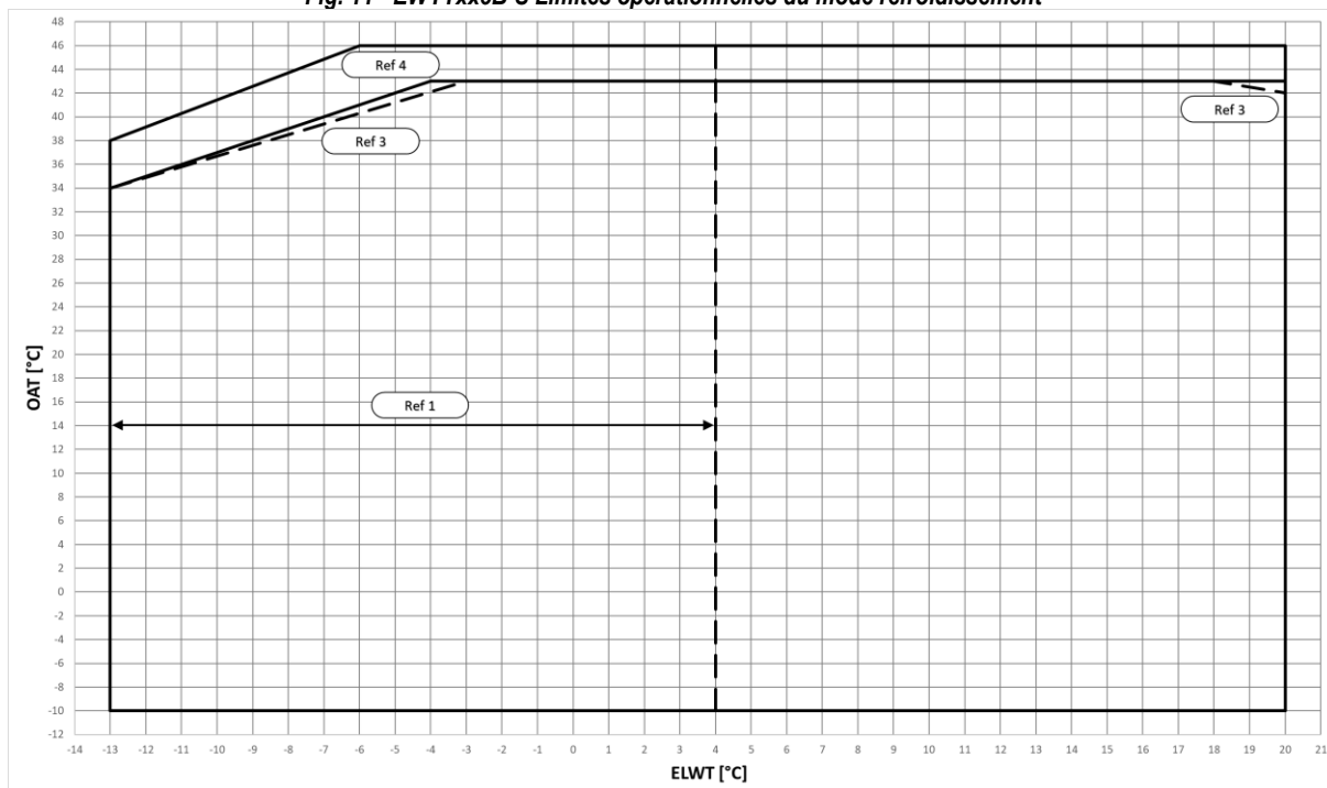
Fig. 12 - EWYTx5B-X Limites opérationnelles du mode refroidissement
