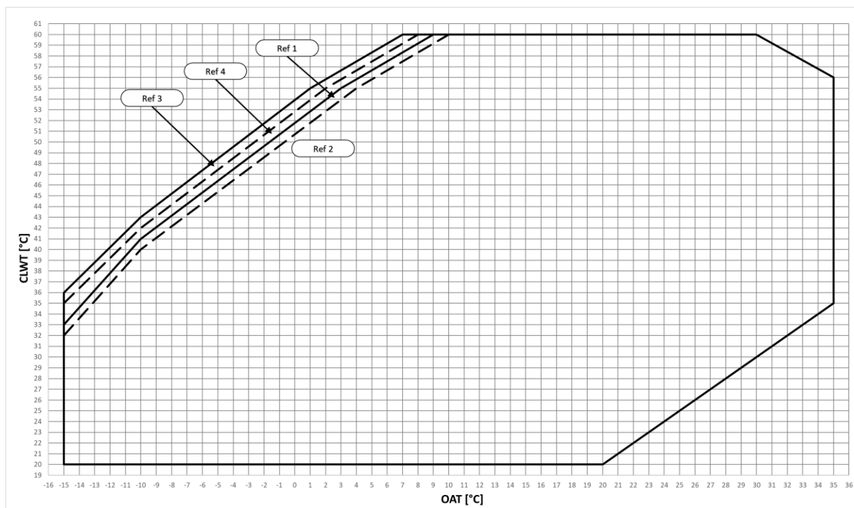
Fig. 15 - EWYT~B-S Limites opérationnelles du mode chauffage
