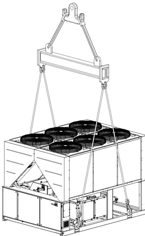
Unité à 4 points de levage
