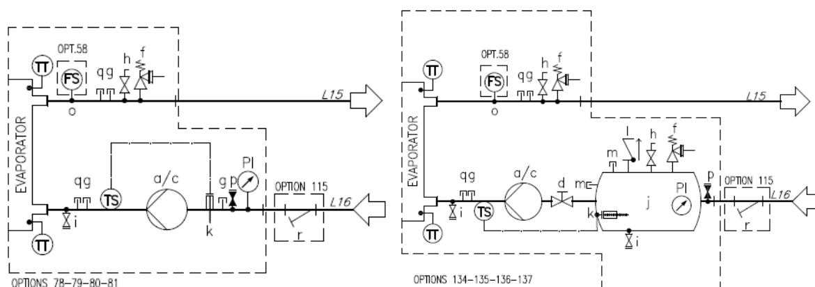
Fig. 10 - Schéma hydraulique pour pompe unique/pompes jumelles (EWATxx0B) (opt. 78-79-80-81/134-135-136-137) (pression de service max. 6 bar)
