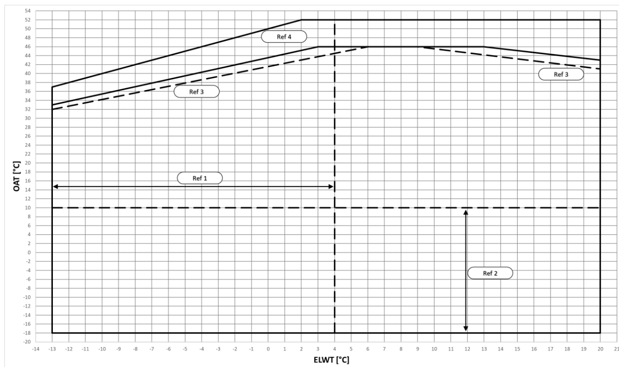
Fig. 13 - EWTxx0B-S Limites opérationnelles du mode refroidissement
