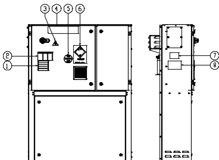
Fig. 20 - Description des étiquettes appliquées sur le tableau électrique EWYTx5B
