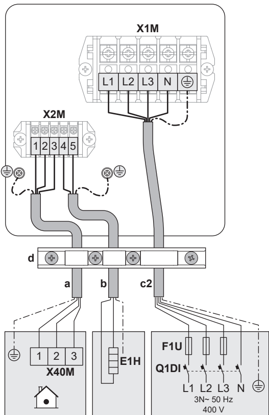
Panoramica del cablaggio: modelli W1 (3N~)
