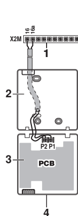
Câblage par l'arrière
