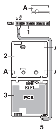
Câblage latéral
