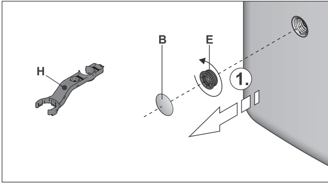
Bild 5-2 Gewindestück herausschrauben
