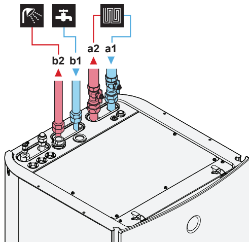
a1 Riscaldamento/raffreddamento ambiente – INGRESSO acqua (collegamento a vite, 1")
