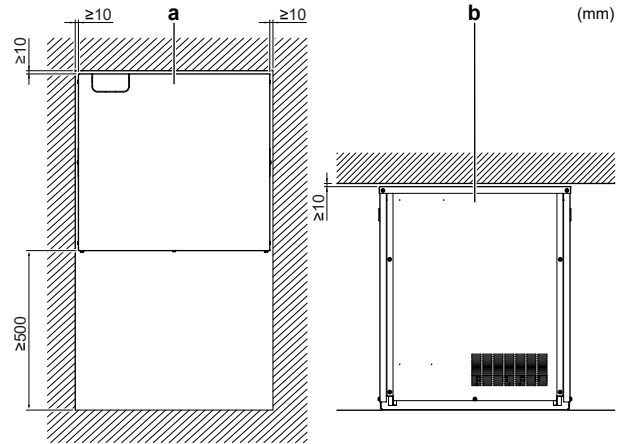
a Vue du dessus b Vue frontale
