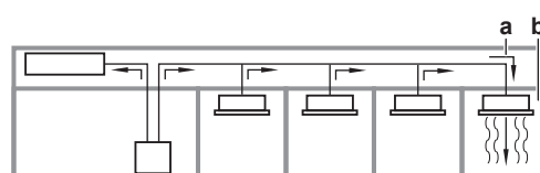
a Richtung des Kältemitteldurchflusses
