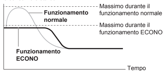
Corrente di funzionamento e consumo elettrico
